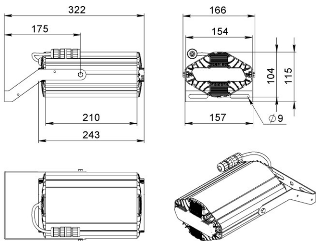
Рисунок 2 Светильник «L-lego II 30 banner» Поворотное крепление
