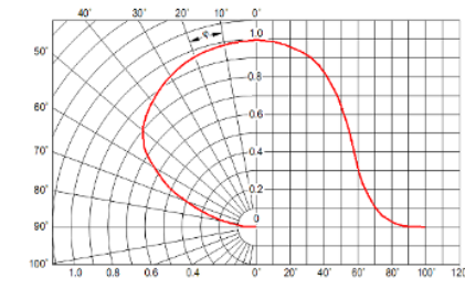
Рисунок 4 Типы КСС
