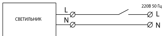
Рисунок 2 Схема подключения светильника «L-office 32»
